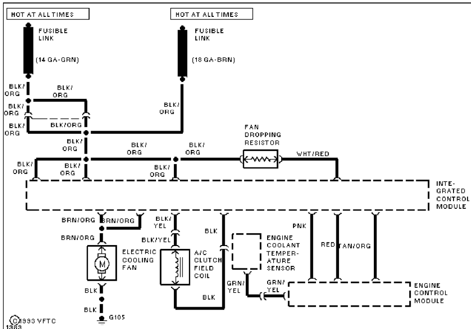
Fig. 19: Cooling Fan Circuit (3.0L SHO)
