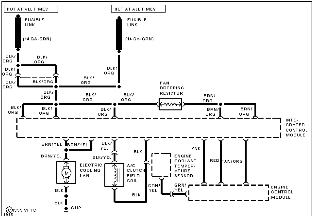
Fig. 17: Cooling Fan Circuit (2.5L)
