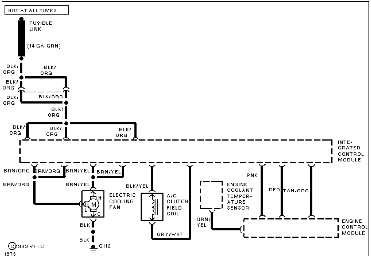
Fig. 20: Cooling Fan Circuit (3.8L)
