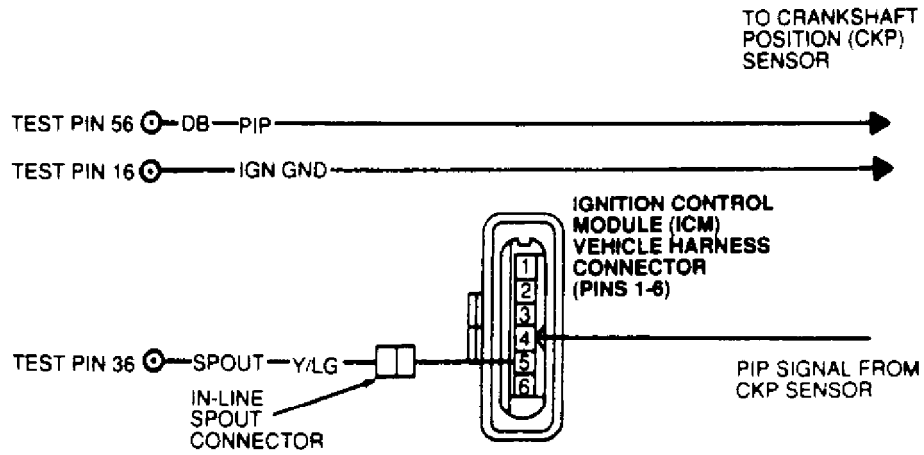
Fig. 131: DIS Module Wiring Harness Connector Terminals (3.2L SHO)
