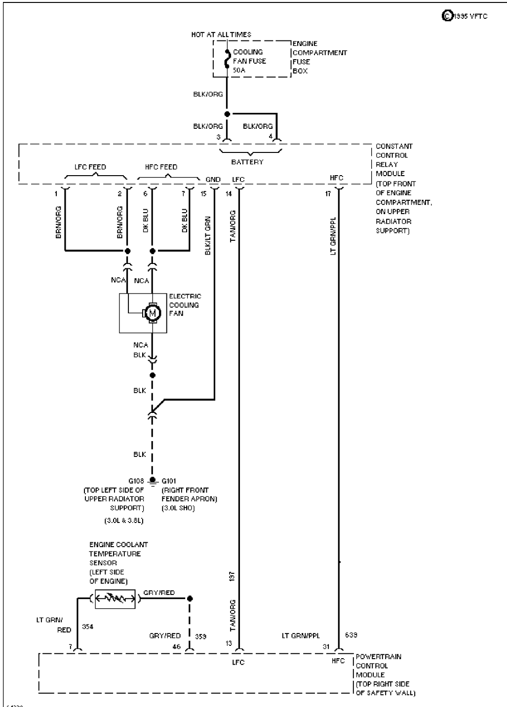
3.0L Flex Fuel, Cooling Fan Circuit
