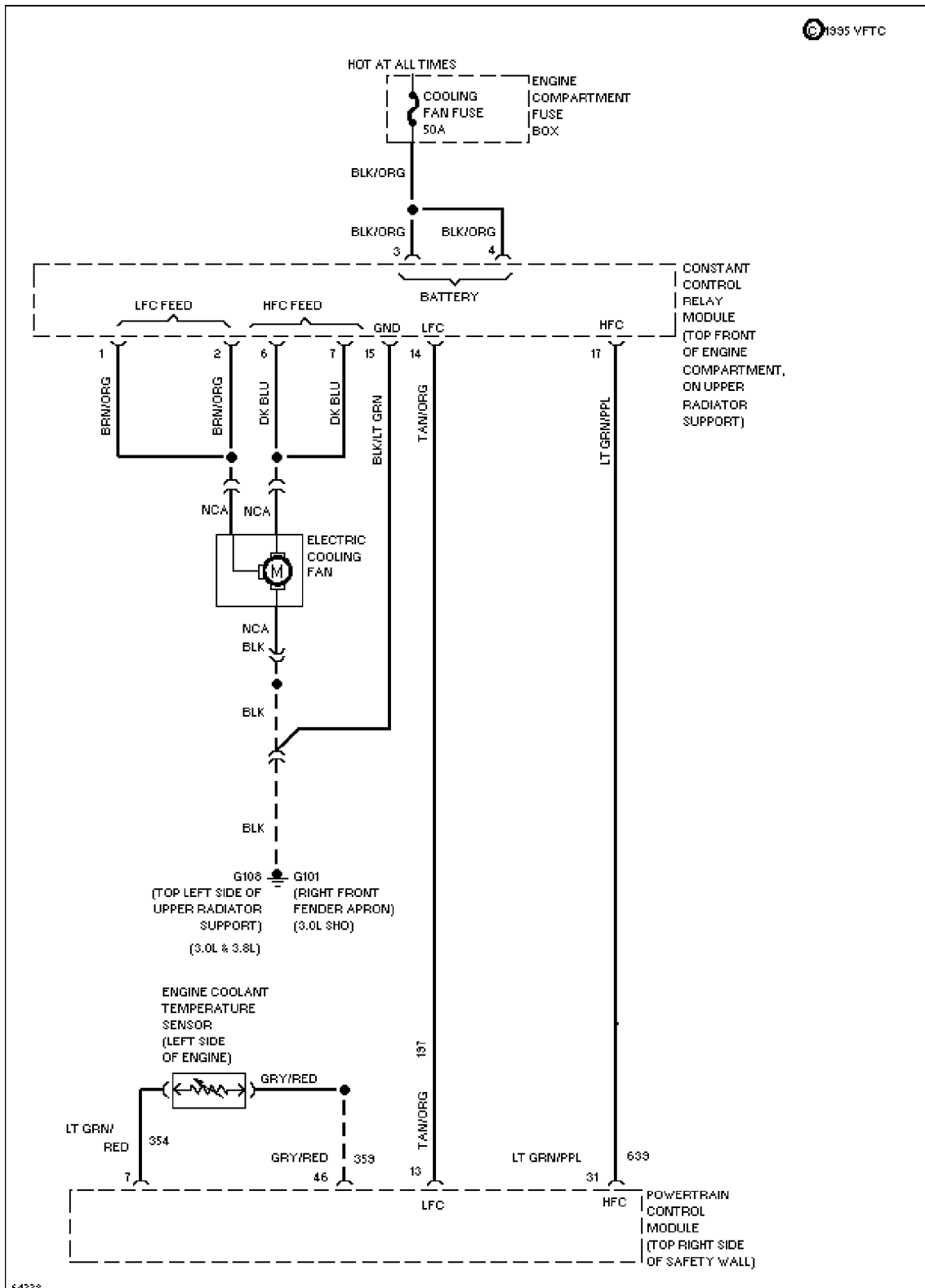
3.0L SHO, Cooling Fan Circuit
