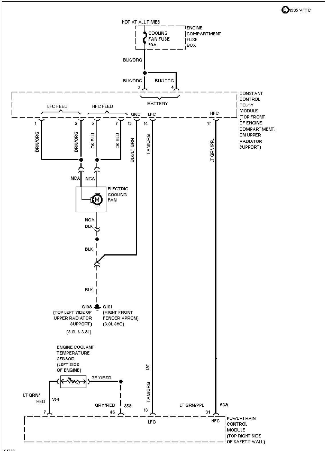
3.0L, Cooling Fan Circuit
