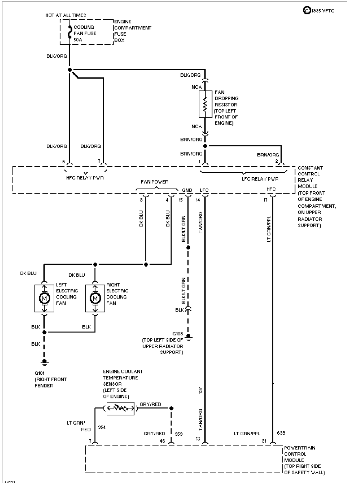
3.2L SHO, Cooling Fan Circuit
