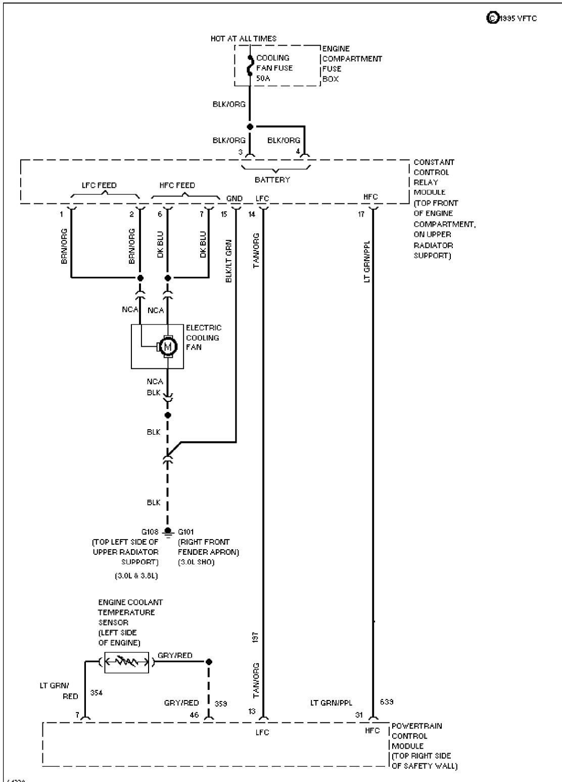
3.8L, Cooling Fan Circuit
